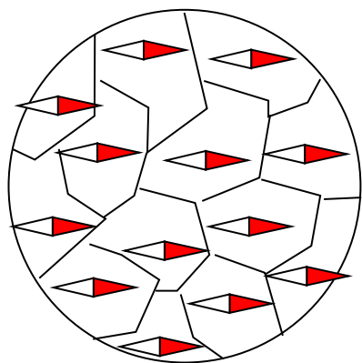
異方性磁粉とその結晶粒
